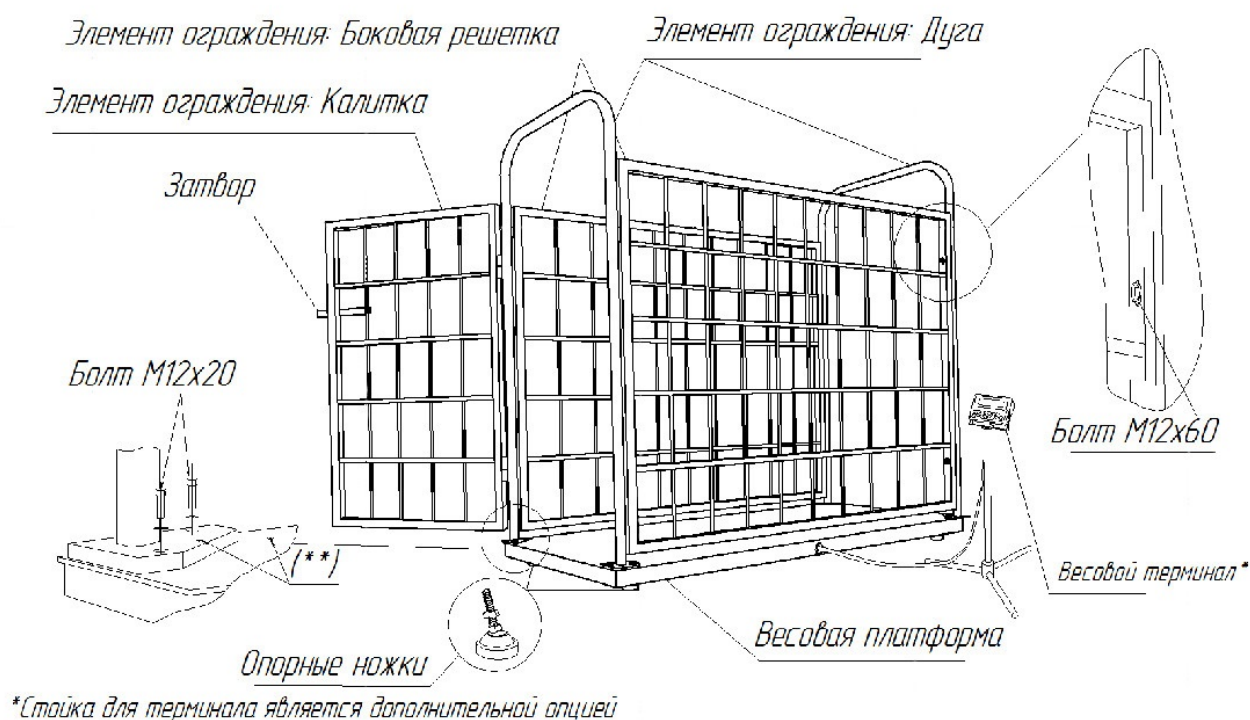
Рисунок – Сборка животноводческих весов «Эльтон»
