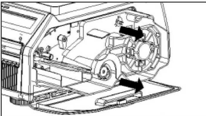
Рисунок 1.15 – Снятие картриджа
