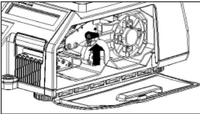
Рисунок 1.14 – Подъем рычага
